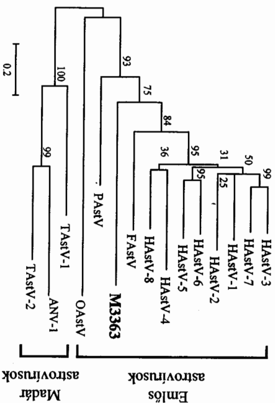
5. ábra "Neighbor-joining filogram" (K2P model, bootstrap 1000-szer) ORF2 régióban (843 nt). Az analízis tartalmazza M3363-et, nyolc humán astrovírus referencia törzset (HAstV-1-től 8-ig) és az állati astrovírusokat: macska (FAstV), sertés (PAstV), bárány (OAsTV) és pulyka astrovírusok: TAsTV-1 and 2, illetve az avian nephritis vírust (ANV-1). A bootstrap értékek az elágazásokban láthatók.
