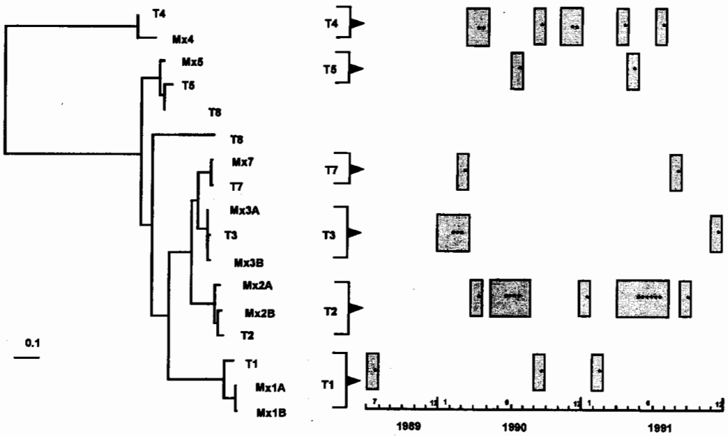
3. ábra Maximum likelihood filogram a referencia törzsek (T1-8) és a mexikói izolátumok szekvenciáinak analízise alapján. (363 bp) Az elágazási pontok szignifikánsak. ( P < 0.05 ) Jobb oldalon látható a típusok előfordulási gyakorisága a tanulmány ideje alatt. Az izolátumok számát csillagok jelzik a szürke mezőben. Mx: Mexikói izolátumok szubtypusai
